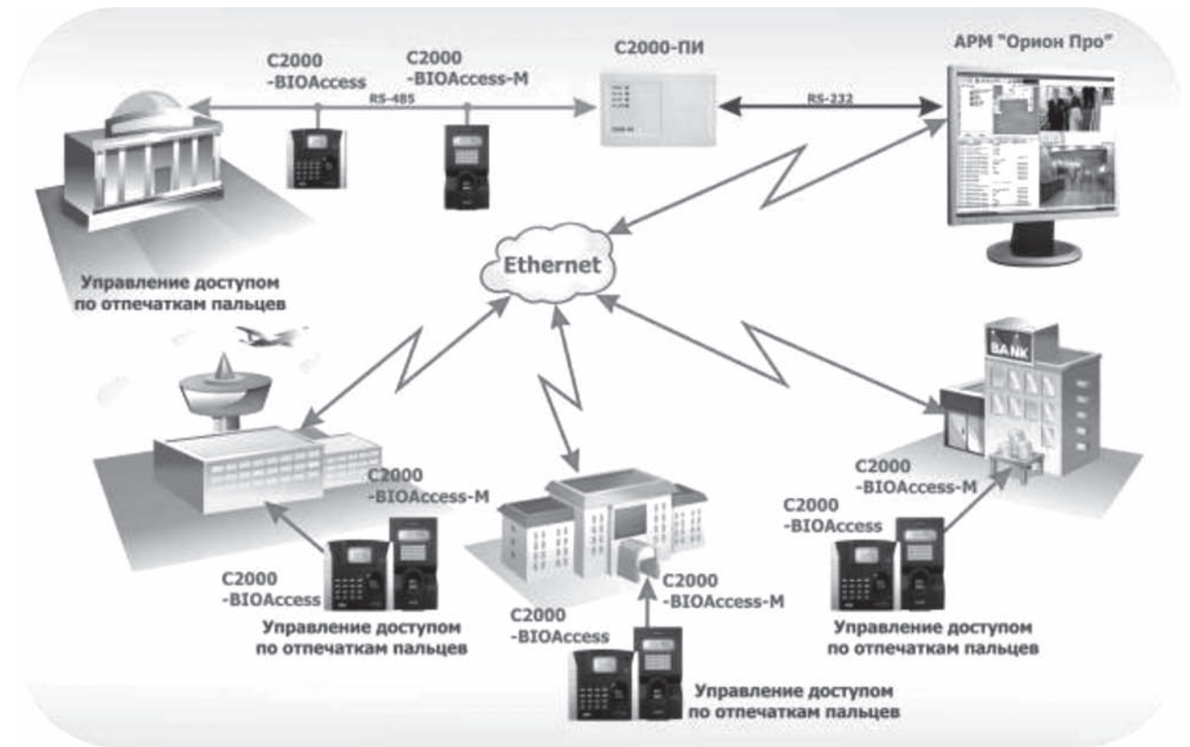
Рис. 4. Подключение биометрических контроллеров к ИСО «ОРИОН»
